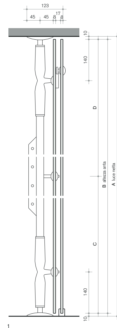
1. sezione verticale 2. sezione orizzontale scorrevole su parete Osso 3. sezione orizzontale scorrevole su muro
